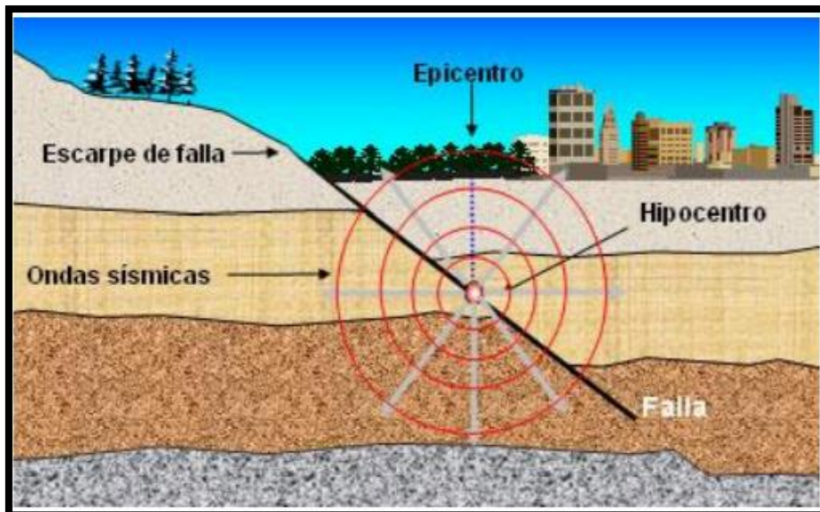
Gráfico N° 19: Sismos originados por una falla geológica.
