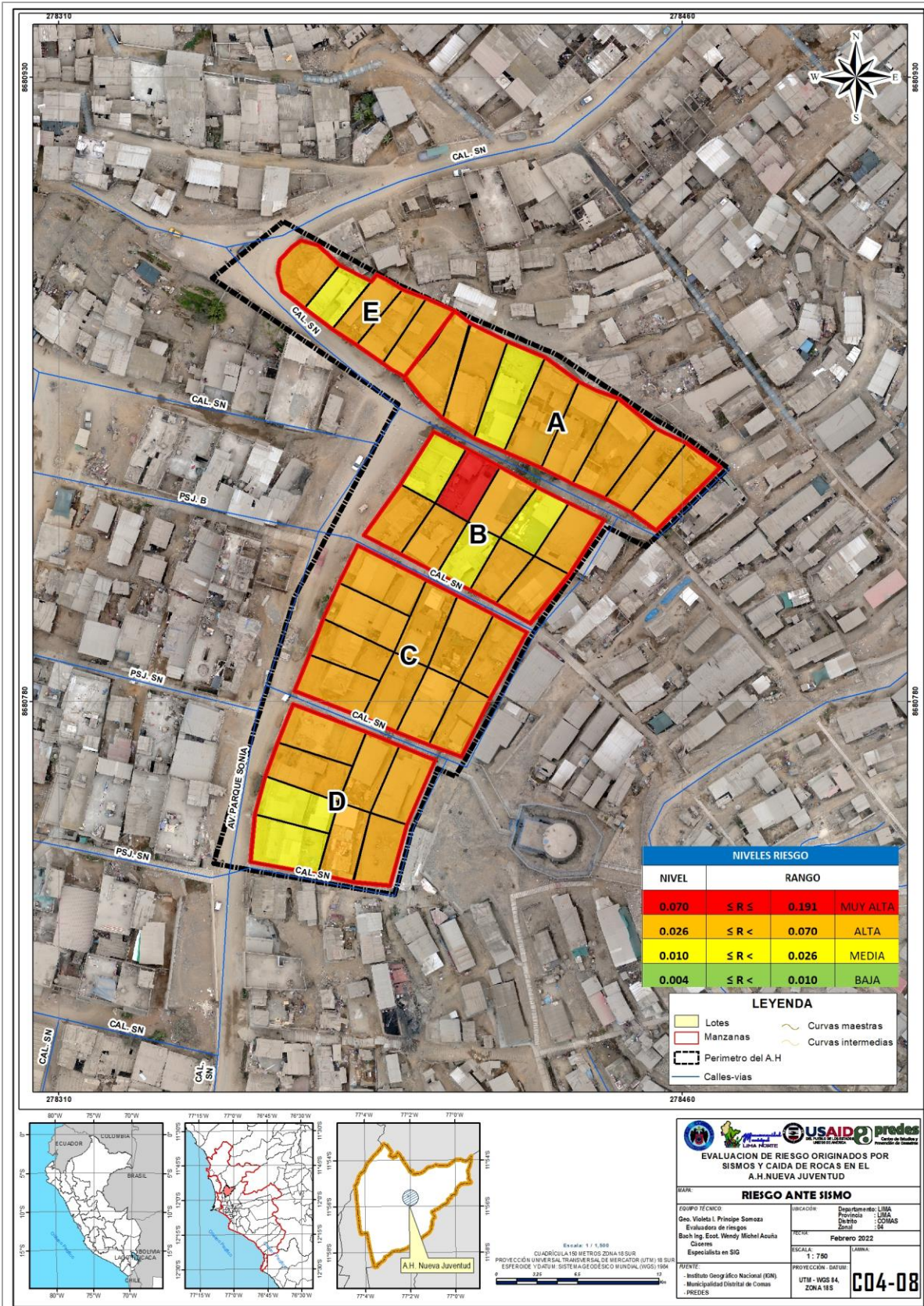
Mapa N° 9: Riesgo por Sismos
