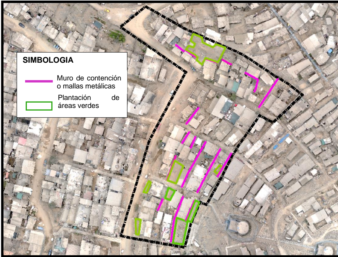
Gráfico N° 24: Propuesta de Medidas Estructurales en el A.H. Nueva Juventud.
