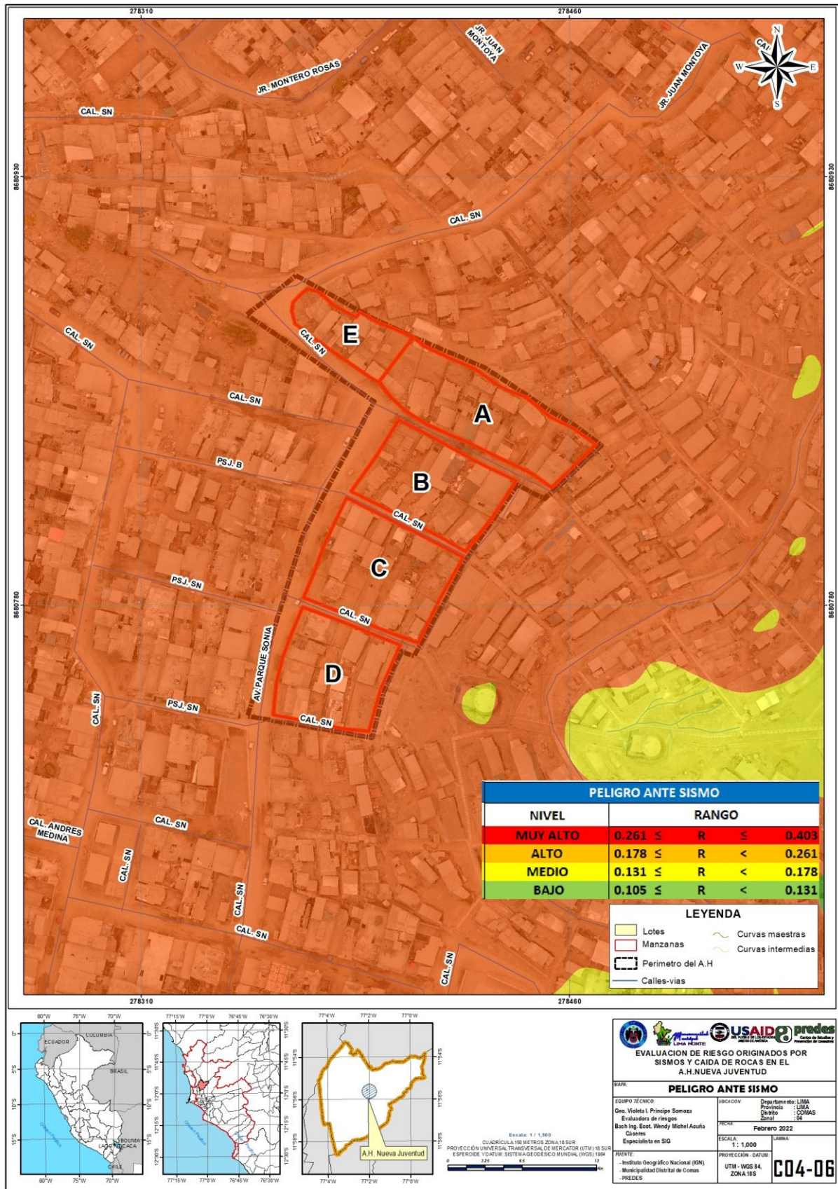
Mapa N°6: Peligro por sismos
