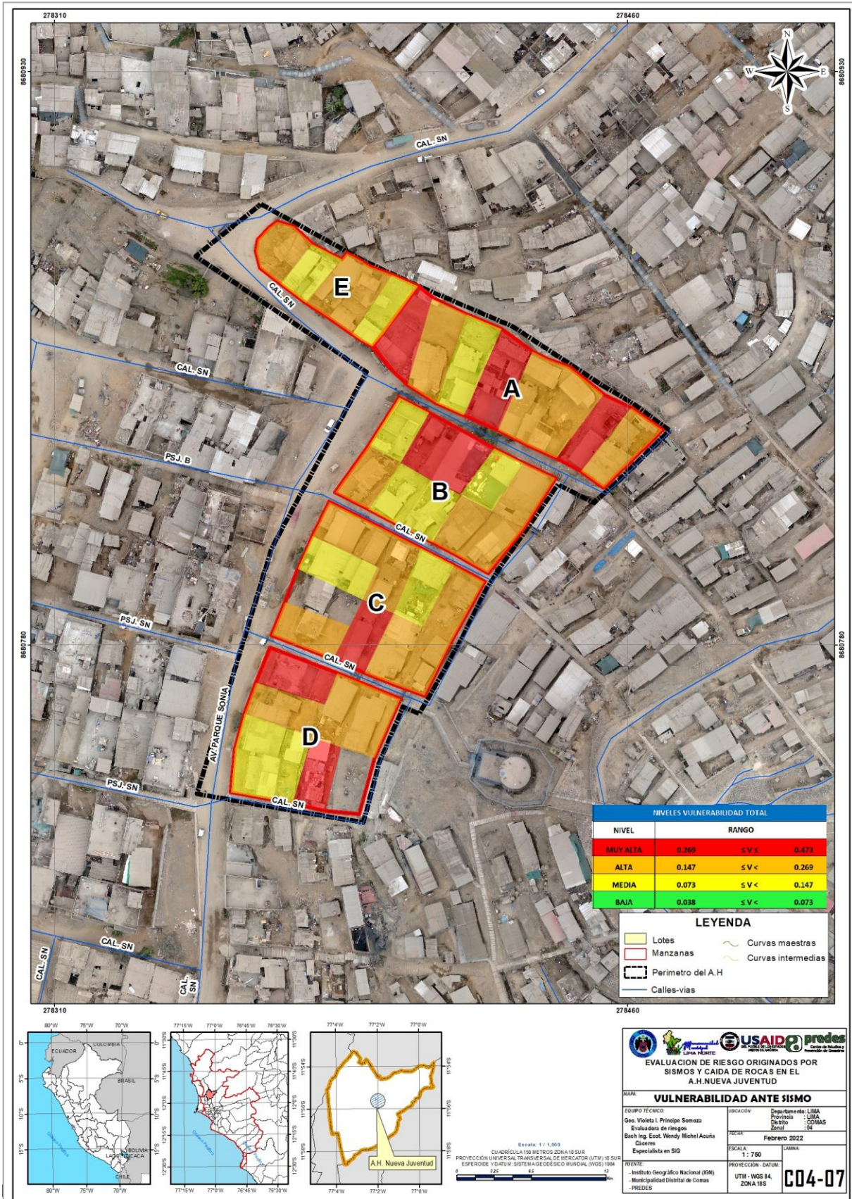
Mapa N° 8: Vulnerabilidad ante Sismos.
