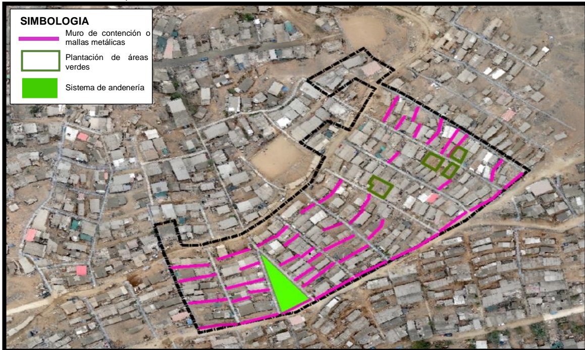
Gráfico N° 29: Propuesta de Medidas Estructurales en el A.H. Próceres Parte Alta la Libertad Zonal II.
