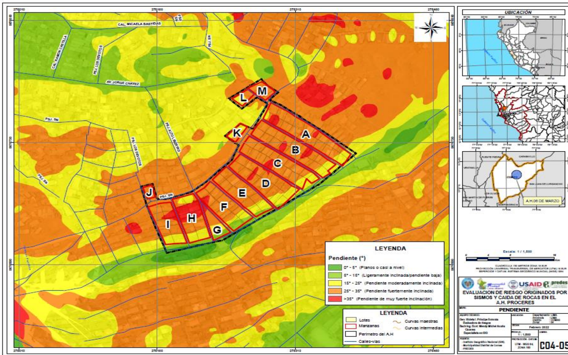
Mapa N° 4: Pendientes
