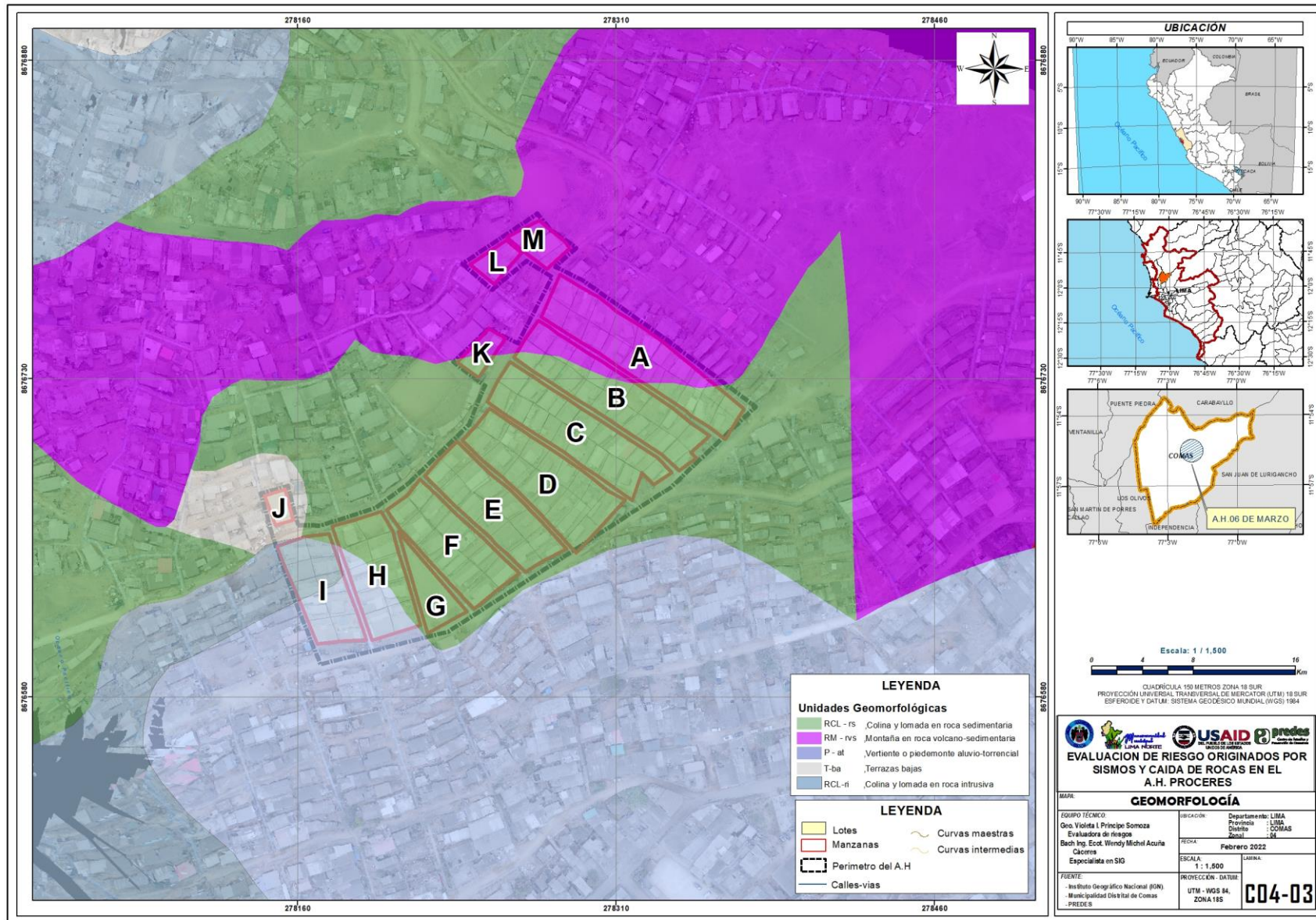
Mapa N° 3: Unidades Geomorfológicas
