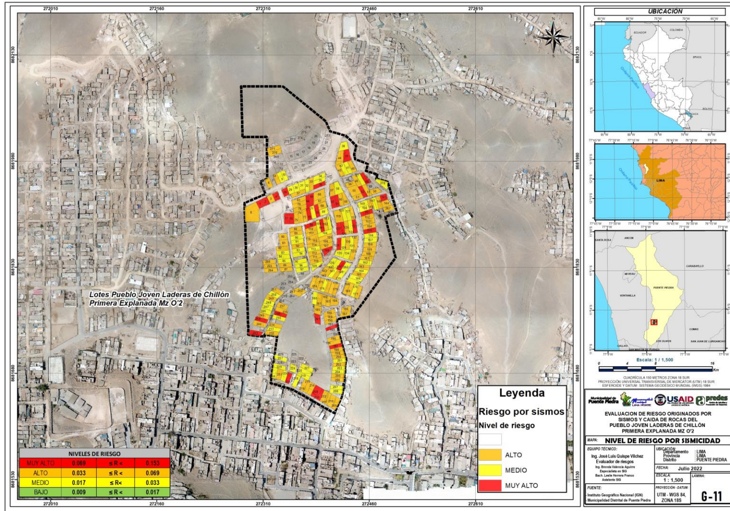
Mapa 23: Mapa de Riesgo por Sismo
