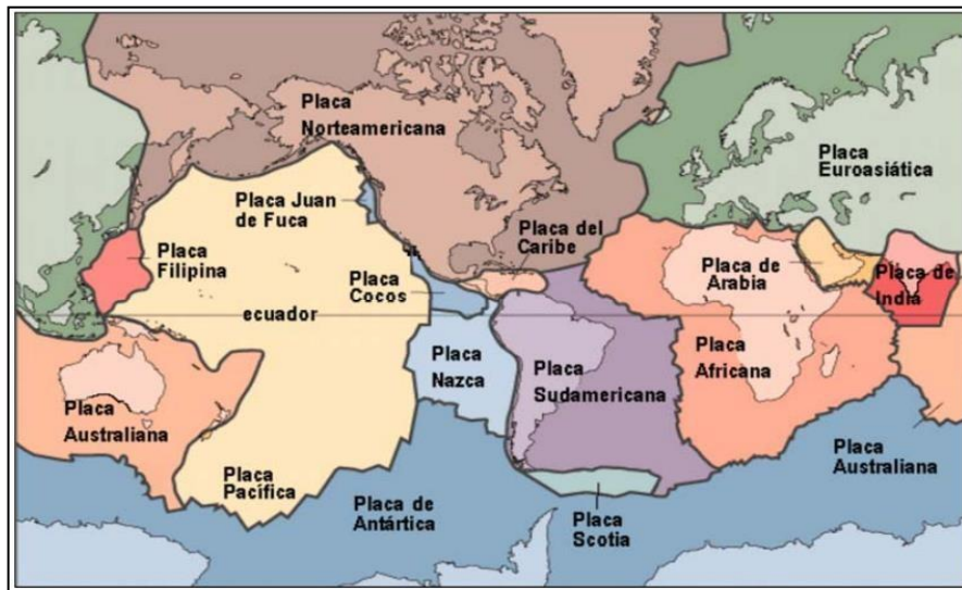
Grafico N° 2. Principales placas tectónicas de la tierra
