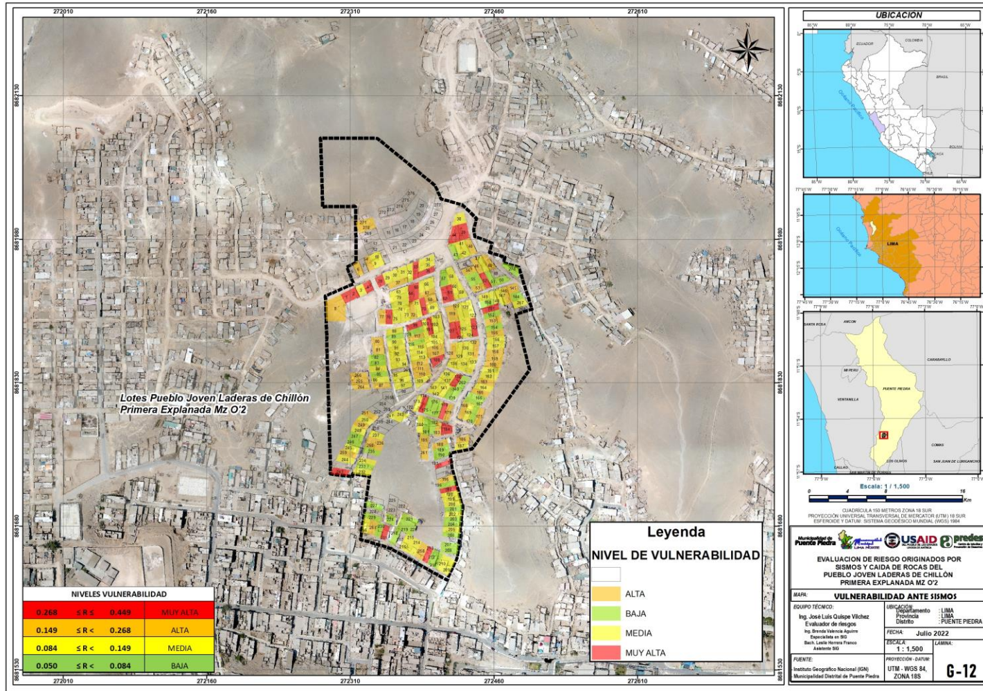
Mapa 21: Mapa de Vulnerabilidad ante sismos
