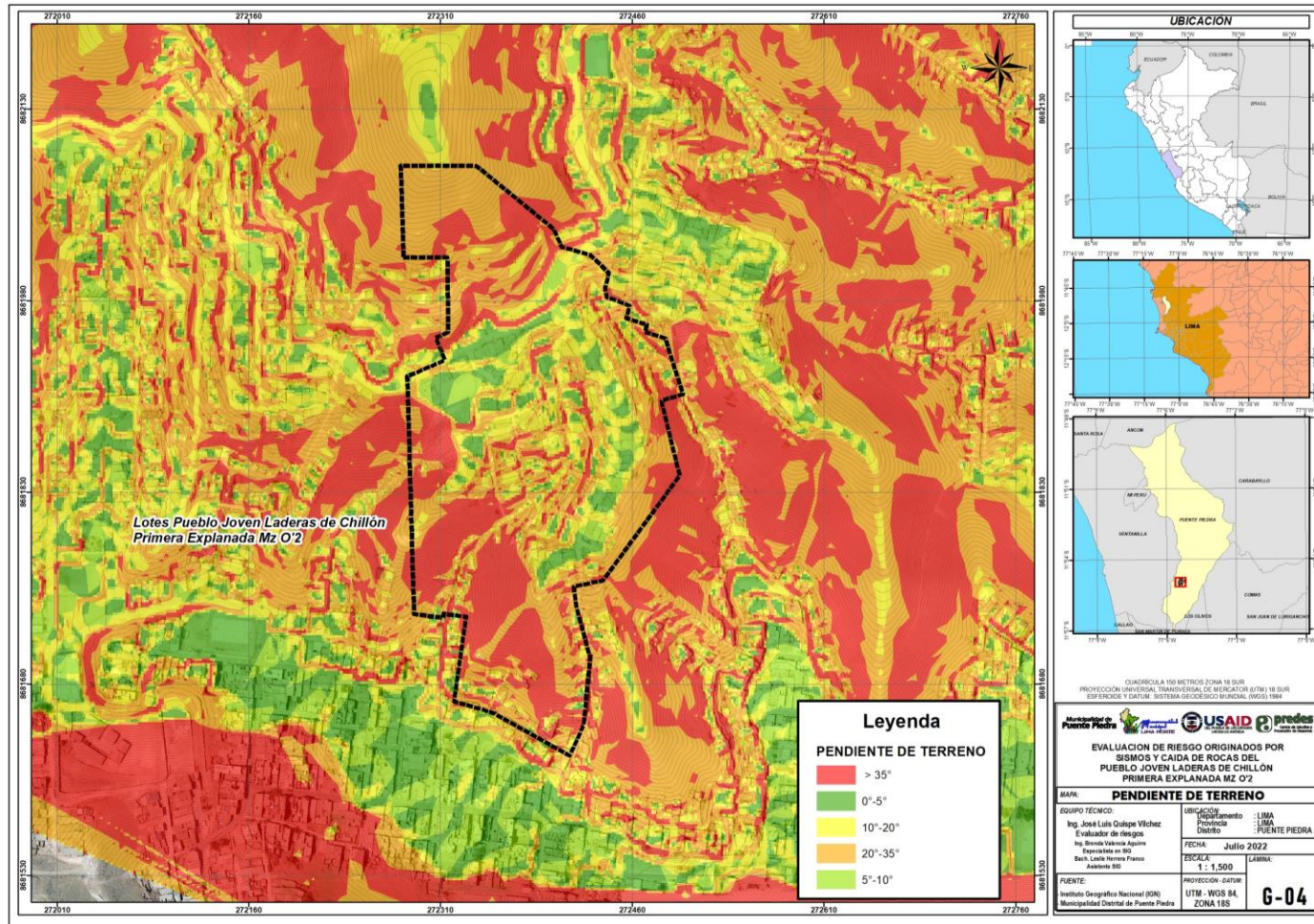
Mapa N° 12. Mapa de Pendiente Pueblo Joven Laderas de Chillón Primera Explanada Mz. O'2 del distrito de Puente Piedra, provincia de Lima, departamento de Lima
