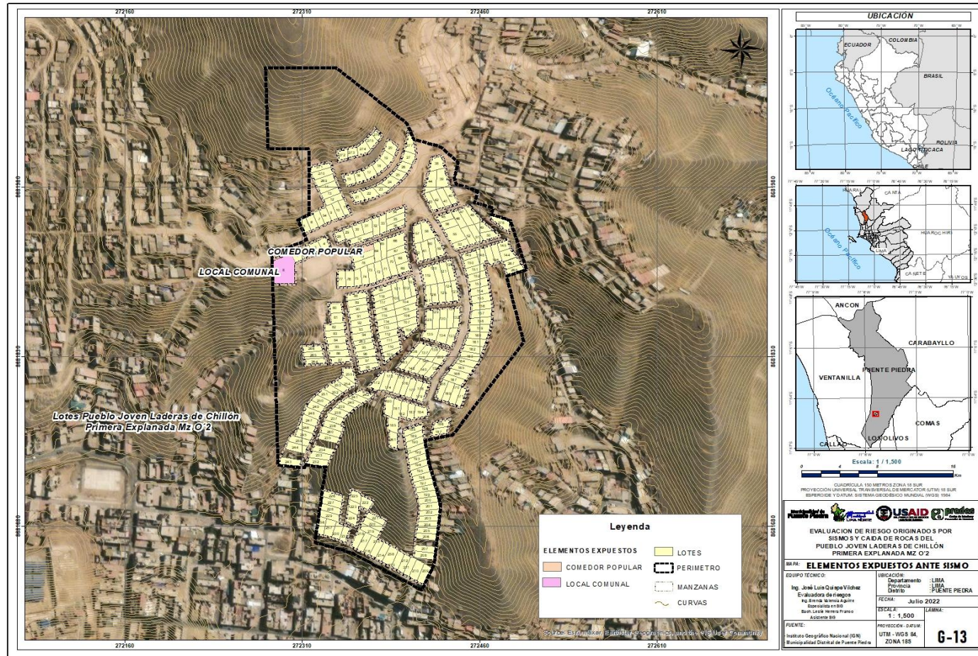
Mapa N° 16. Mapa de Elementos expuestos ante sismo del Pueblo Joven Laderas de Chillón Primera Explanada Mz. O'2, del distrito de Puente Piedra, provincia de Lima, departamento de Lima
