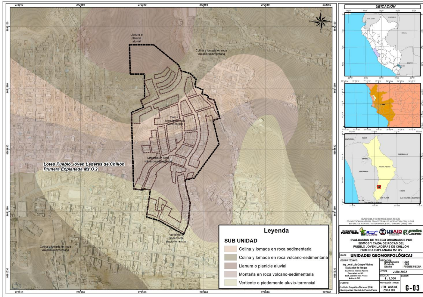
Mapa N° 9. Mapa Geomorfológico Pueblo Joven Laderas de Chillón Primera Explanada Mz. O'2 del distrito de Puente Piedra, provincia de Lima, departamento de Lima
