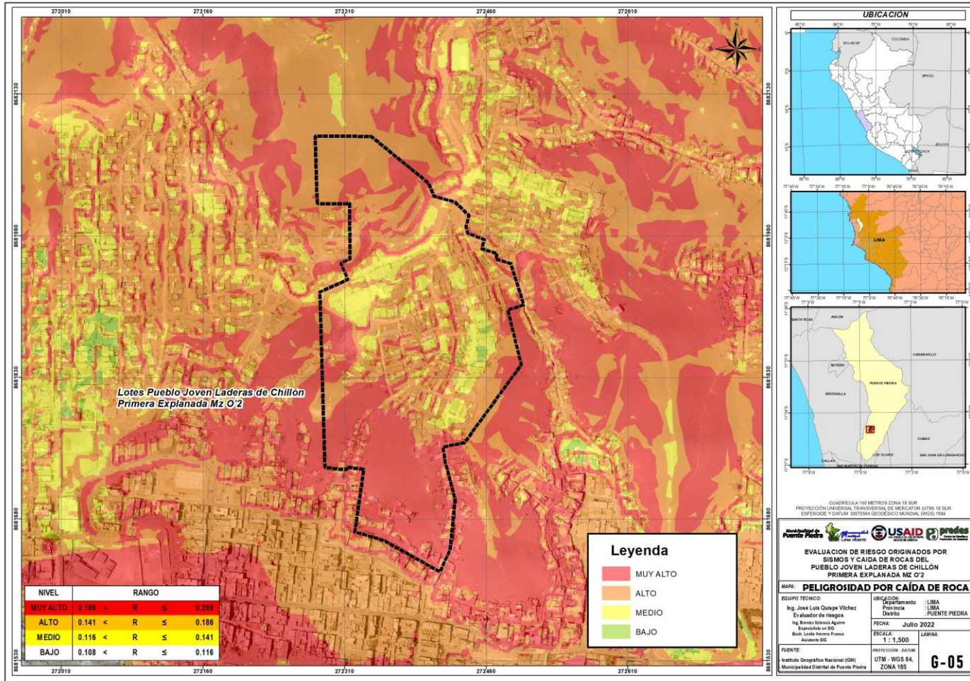
Mapa N°18. Mapa de Peligro por Caída de Rocas Pueblo Joven Laderas de Chillón Primera Explanada Mz. O'2, del distrito de Puente Piedra, provincia de Lima, departamento de Lima
