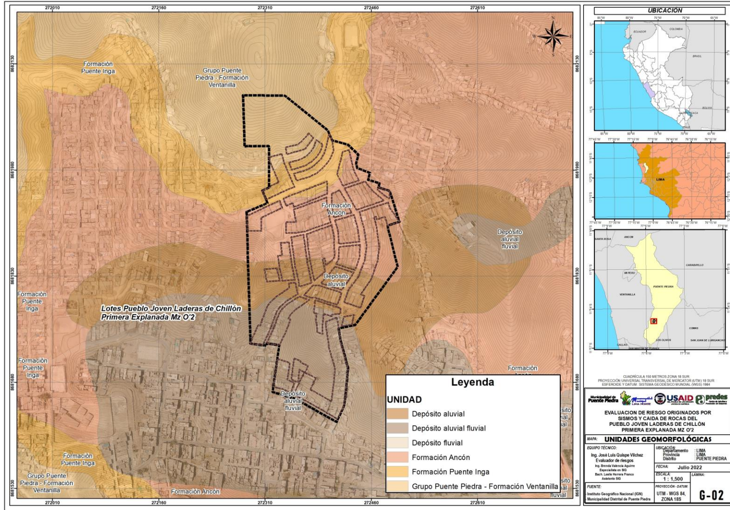
Mapa N° 8. Mapa Geológico Pueblo Joven Laderas de Chillón Primera Explanada Mz. O'2, del distrito de Puente Piedra, provincia de Lima, departamento de Lima
