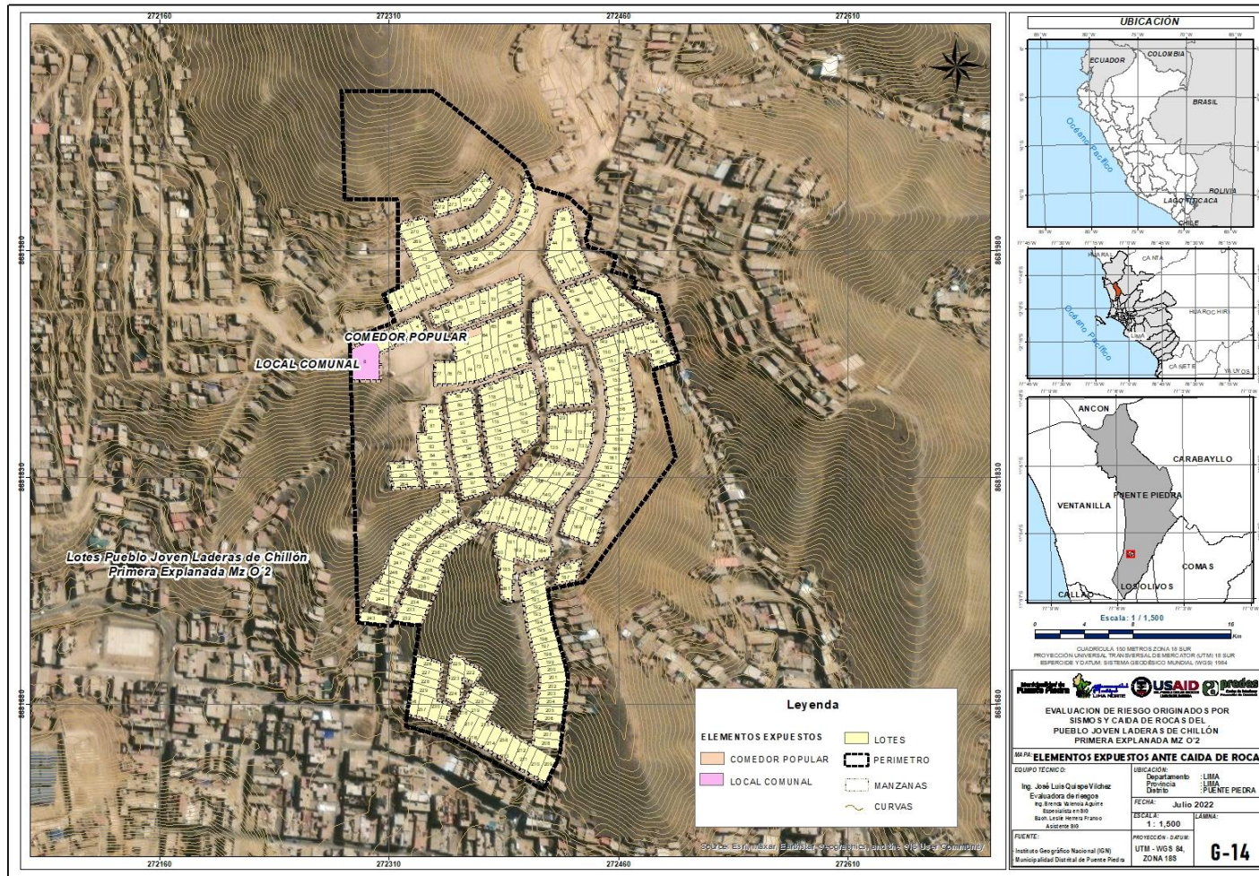
Mapa N° 17. Mapa de Elementos expuestos ante caída de rocas del Pueblo Joven Laderas de Chillón Primera Explanada Mz. O'2, del distrito de Puente Piedra, provincia de Lima, departamento de Lima
