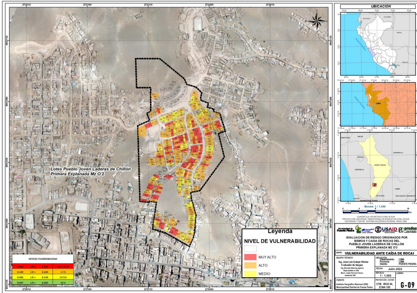
Mapa 20: Mapa de Vulnerabilidad ante caídas de rocas
