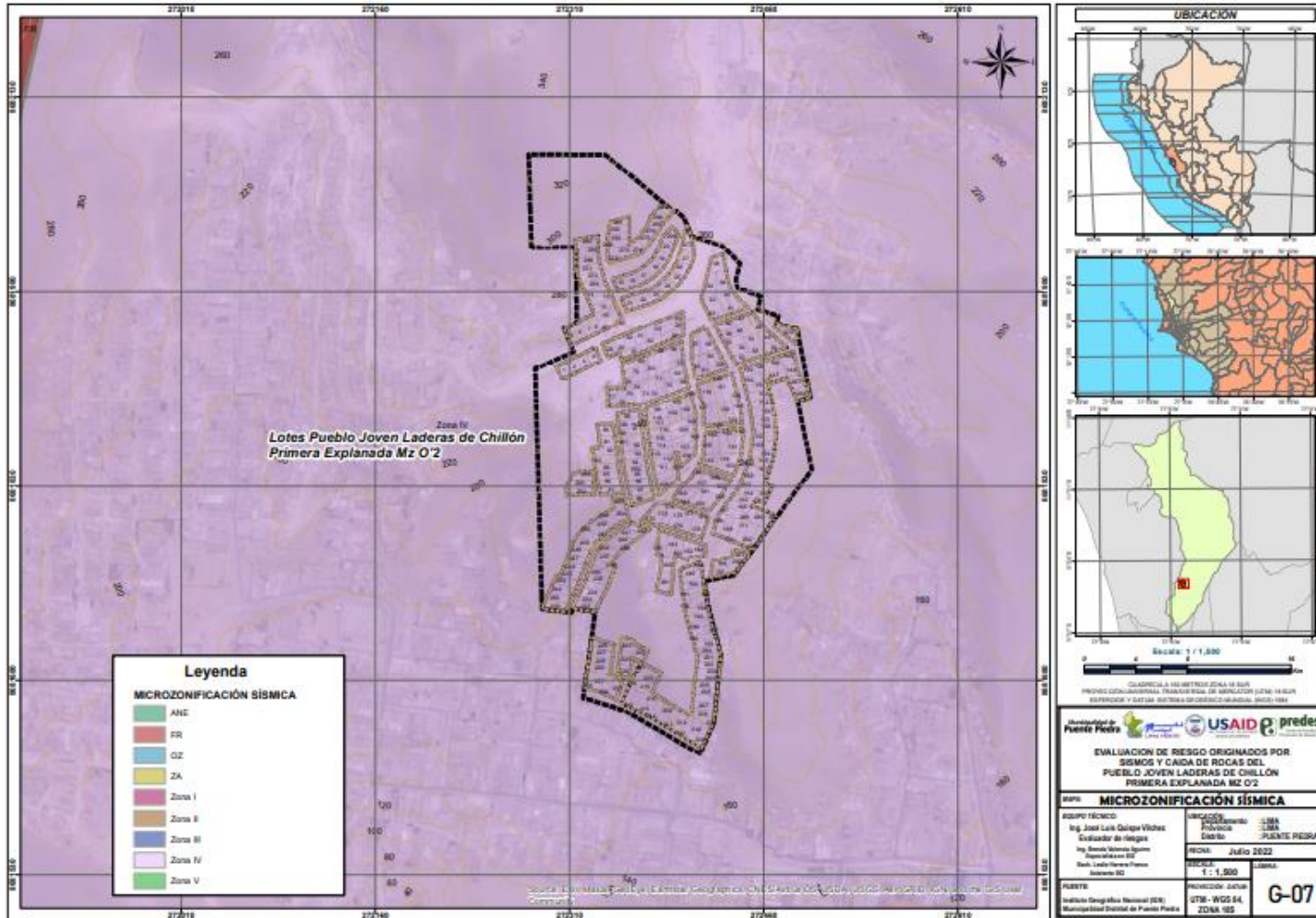
Mapa N° 10. Mapa de Microzonificación Sísmica Pueblo Joven Laderas de Chillón Primera Explanada Mz. O'2, del distrito de Puente Piedra, provincia de Lima, departamento de Lima
