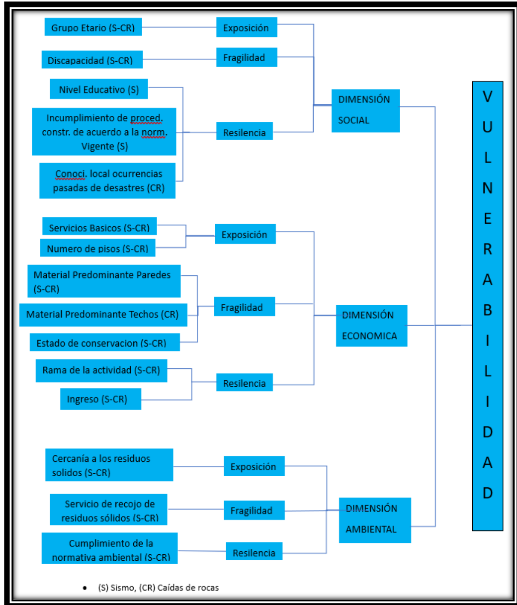
Gráfico N° 13; Flujoograma general del análisis de la vulnerabilidad de Caídas de rocas y de Sismos del área de influencia en el Pueblo Joven Laderas de Chillón Primera Explanada Mz. O'2.
