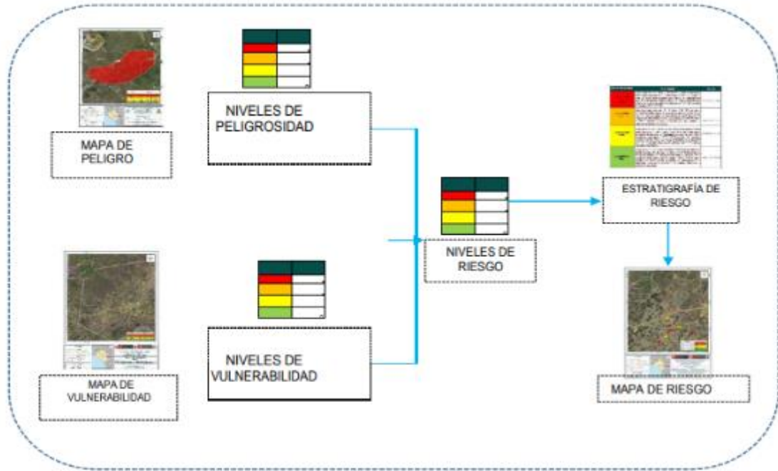
Gráfico 22. Metodología para determinar los niveles del riesgo
