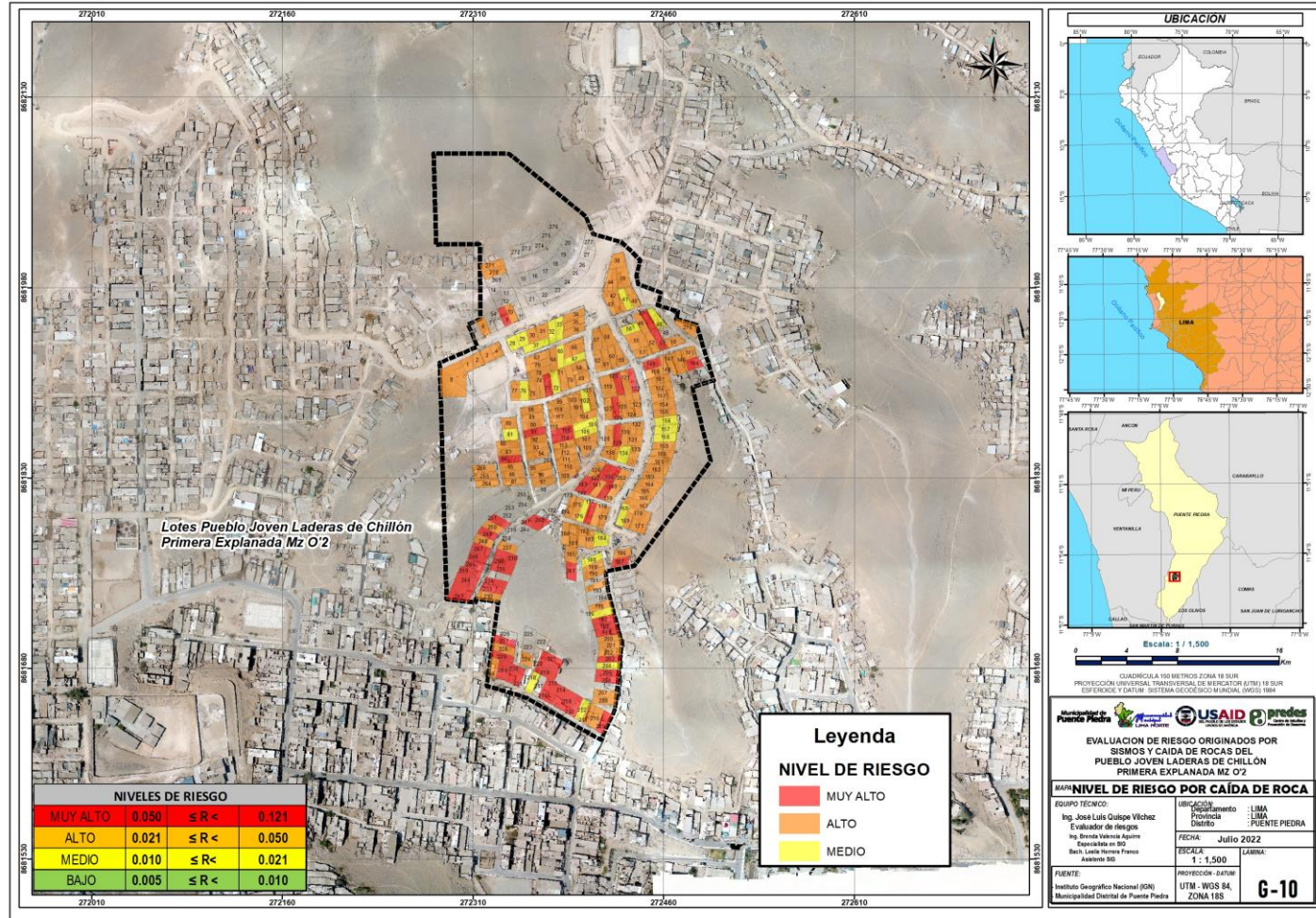
Mapa 22: Mapa de Riesgo por Caída de roca
