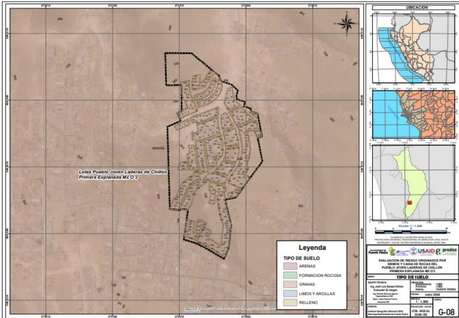
Mapa N° 13. Mapa de Tipo de Suelo de Pueblo Joven Laderas de Chillón Primera Explanada Mz O'2, del distrito de Puente Piedra, prov. de Lima, depart. de Lima
