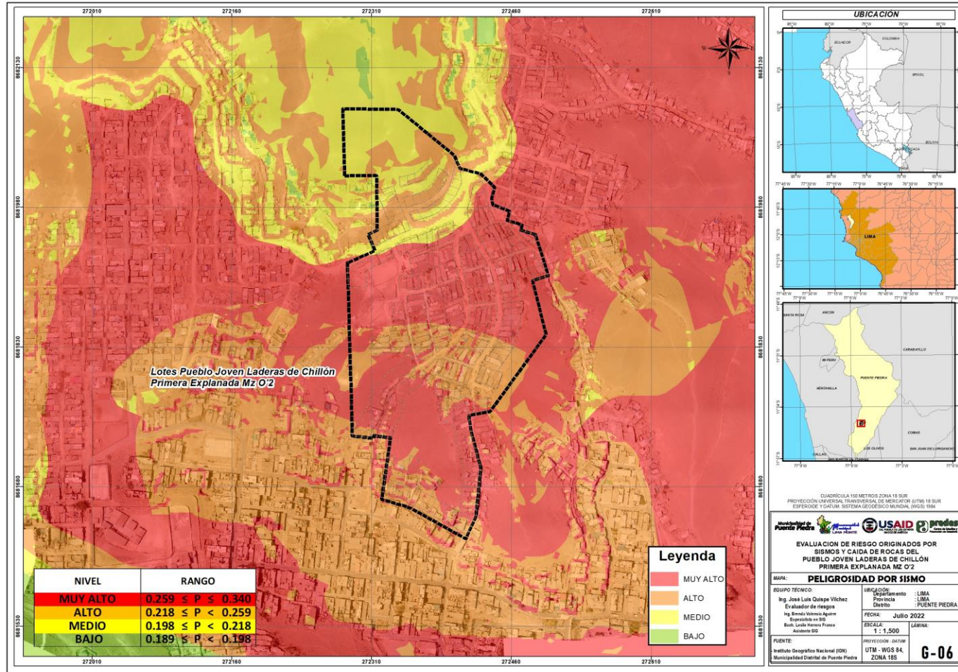
Mapa N° 19. Mapa de Peligro Sísmico de Pueblo Joven Laderas de Chillón Primera Explanada Mz. O'2 del distrito de Puente Piedra, provincia de Lima, departamento de Lima
